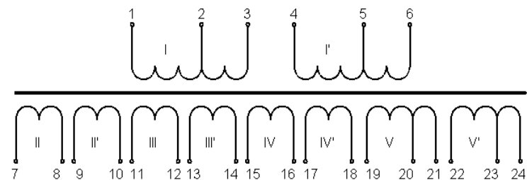
Схема обмоток трансформаторов ТАН
